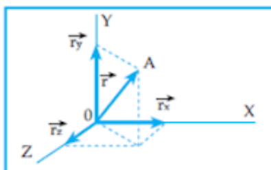
Gambar 1.6 Vektor satuan
